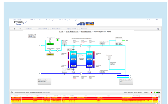
Pufferspeicher Kälte in der Kältetechnik im Ärztehaus
